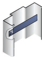
A3 Recessed Metal Stud Anchor
