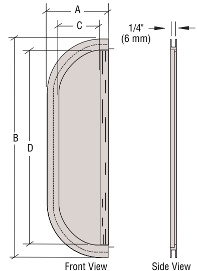
TP125 Template
