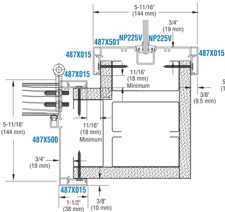
15 Corner Hinge Jamb/Wall Jamb
