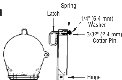
Door Cap Cross Section
