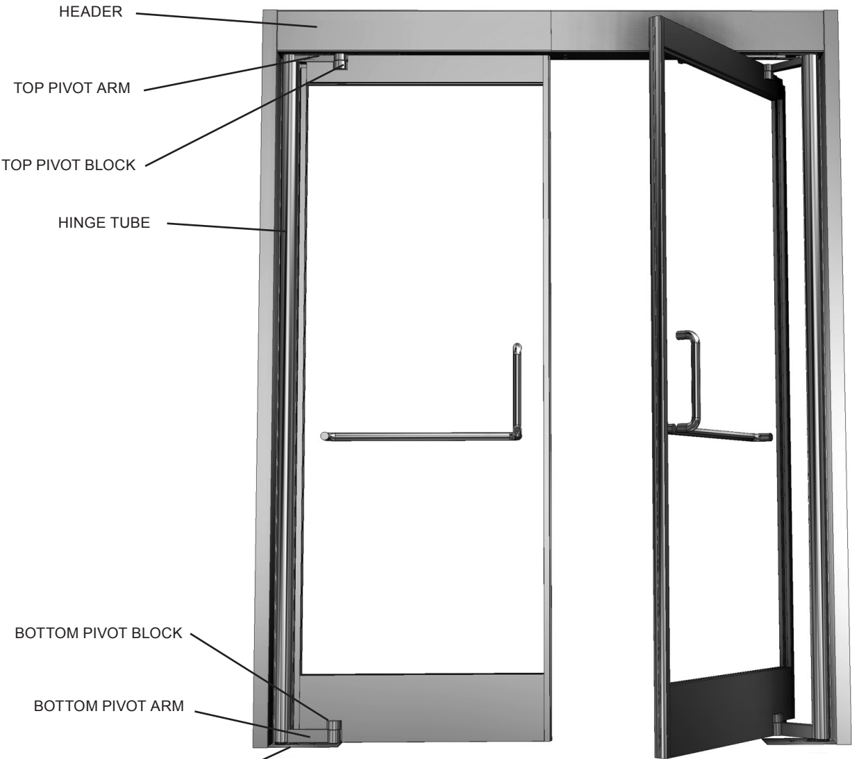
LEFT HAND REVERSE DOOR
