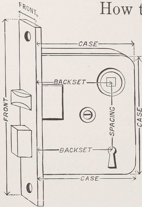
INSIDE DOOR LOCK
