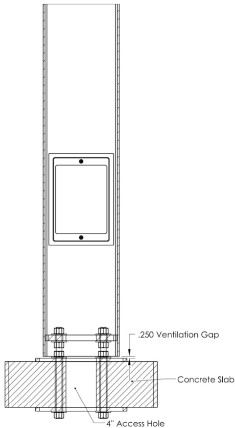
SECTION A-A SCALE 1 : 6
