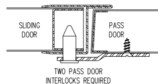
C PASS DOOR INTERLOCK SECTION
