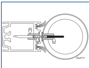
331001912 Cable Door Leaf
