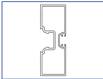
US01-0425-LLCL 4 1/2" Jamb Tube
