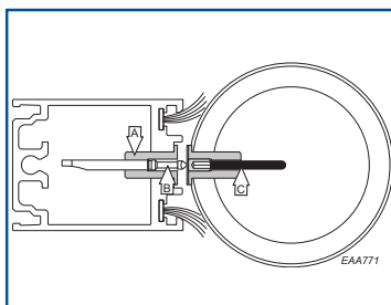
331001913 Cable Door Center Shaft
