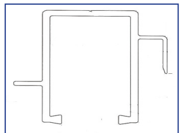
US01-2001-LLMF ICU Track, Mill Finish
