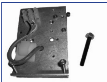
US15-0382-02 Kit, Door Position Switch, RH
