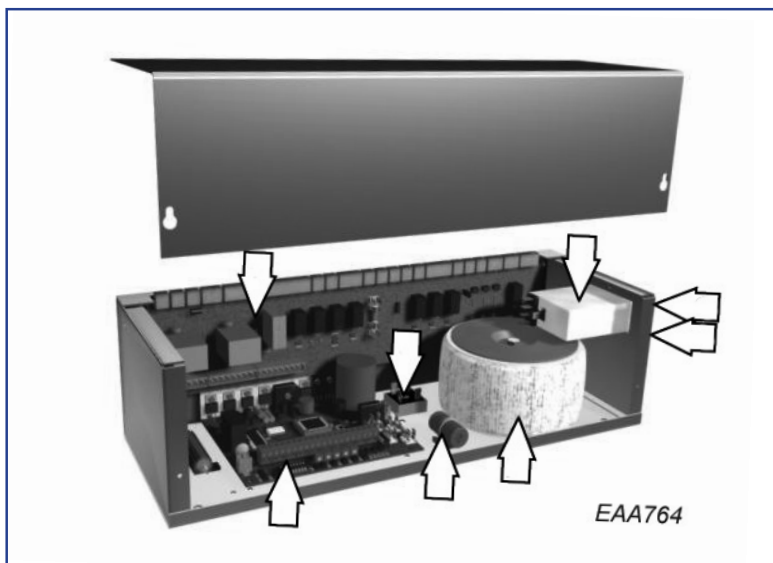
Control Box RD3 / RD4A1
