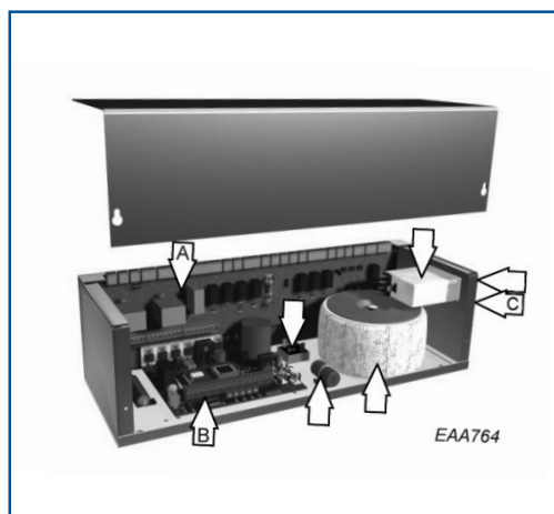
Control Box RD3 / RD4A1
