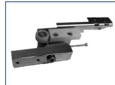
331002121 Door Carriage Top Mid Uniturn w/Slider (D)
