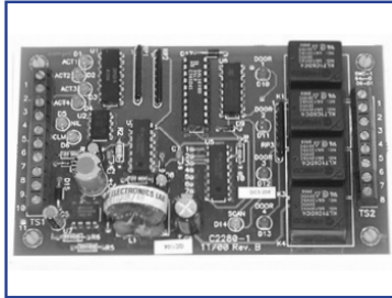
H2280 Module, 4 Door Interlock Control
