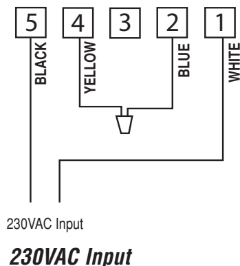
Fig. 3 - 230VAC Input
