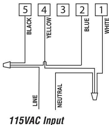
Fig. 2 - 115VAC Input
