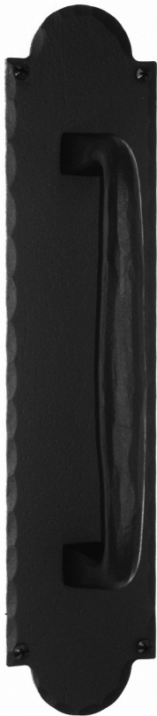
ILQBP 15-3/4" H x 3-1/2" W proj. 4"
