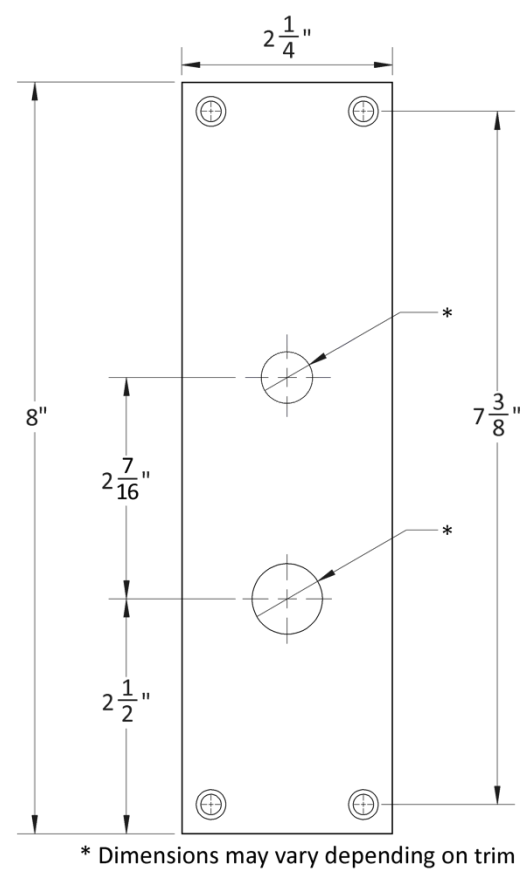
1E-ADA ADA Thumb Turn
