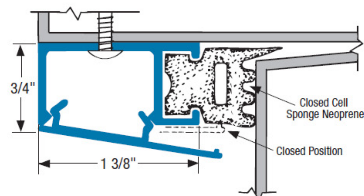
No: 1500* Aluminum
