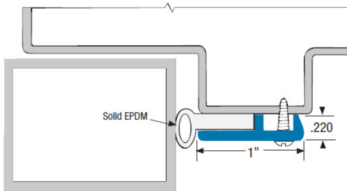
No: 192* Aluminum
