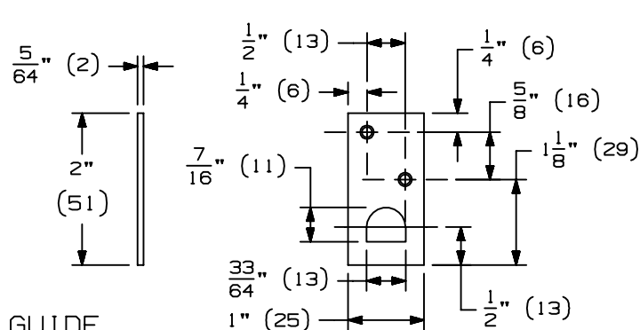
GUIDE
