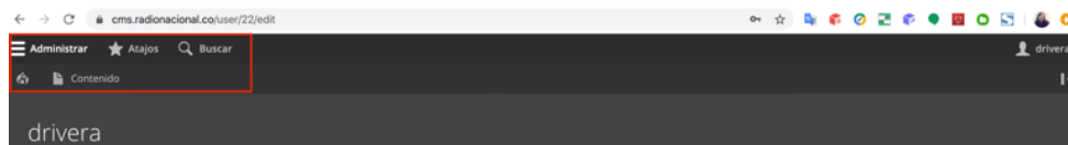
Ilustración 3: Menú Administración
