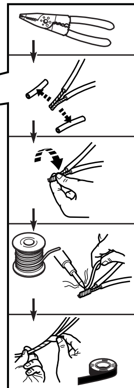
FACTORY INSTALLED 7-WAY TRAILER TOW INSTALLATION EN USINE INSTALACIÓN DE FÁBRICA
