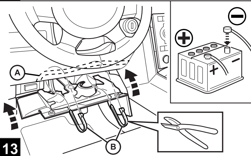
FACTORY INSTALLED 7-WAY TRAILER TOW INSTALLATION EN USINE INSTALACIÓN DE FÁBRICA
