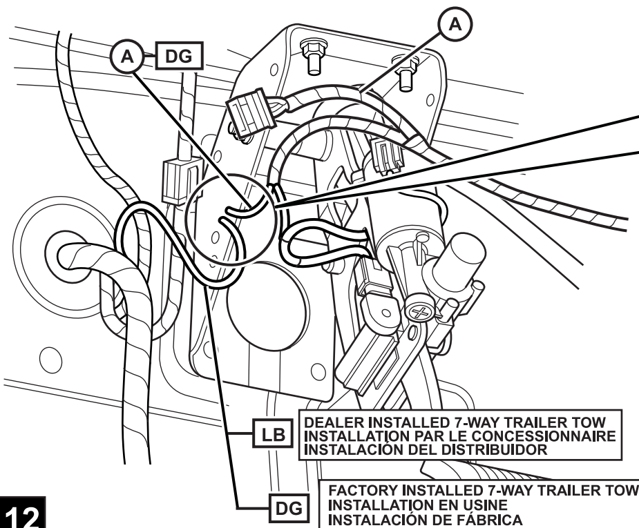
DEALER INSTALLED 7-WAY TRAILER TOW INSTALLATION PAR LE CONCESSIONNAIRE INSTALACIÓN DEL DISTRIBUIDOR
