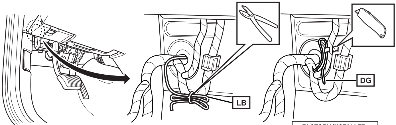
DEALER INSTALLED 7-WAY TRAILER TOW INSTALLATION PAR LE CONCESSIONNAIRE INSTALACIÓN DEL DISTRIBUIDOR
