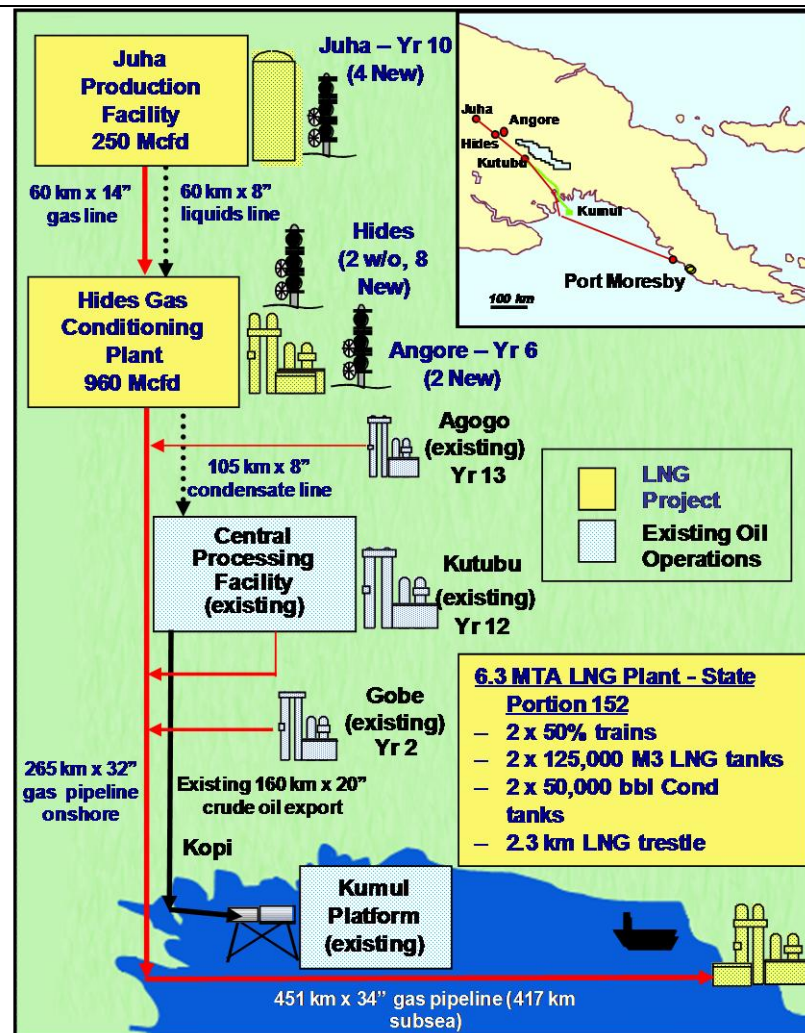
Figure 1 PNG LNG Project Schematic
