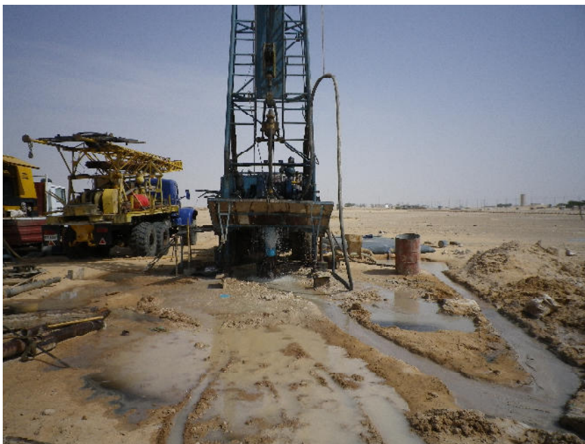
Travaux de forage à Boulénouar
