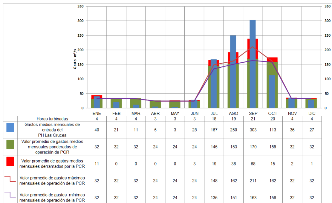
Figura 3. Comparación de caudales medios mensuales actuales en el río San Pedro con los medios mensuales esperados con la operación del PH Las Cruces
