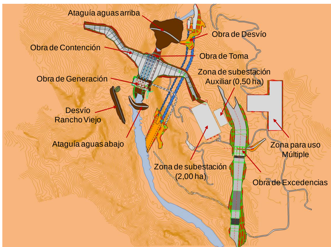
Figura 2. Esquema general de obras para la cortina de CCR
