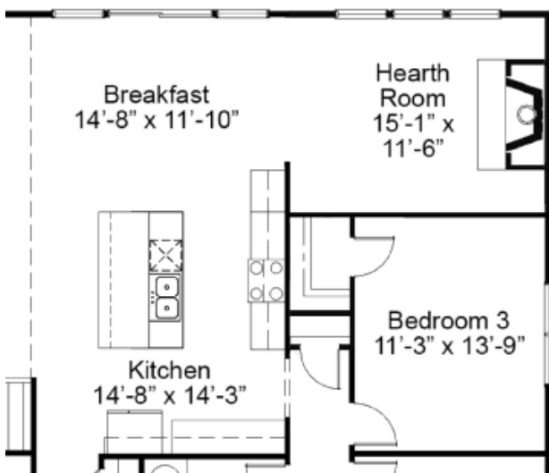
OPTIONAL CORNER HEARTH
