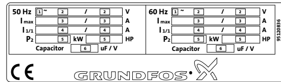
Fig. 2 Plaque signalétique du moteur
