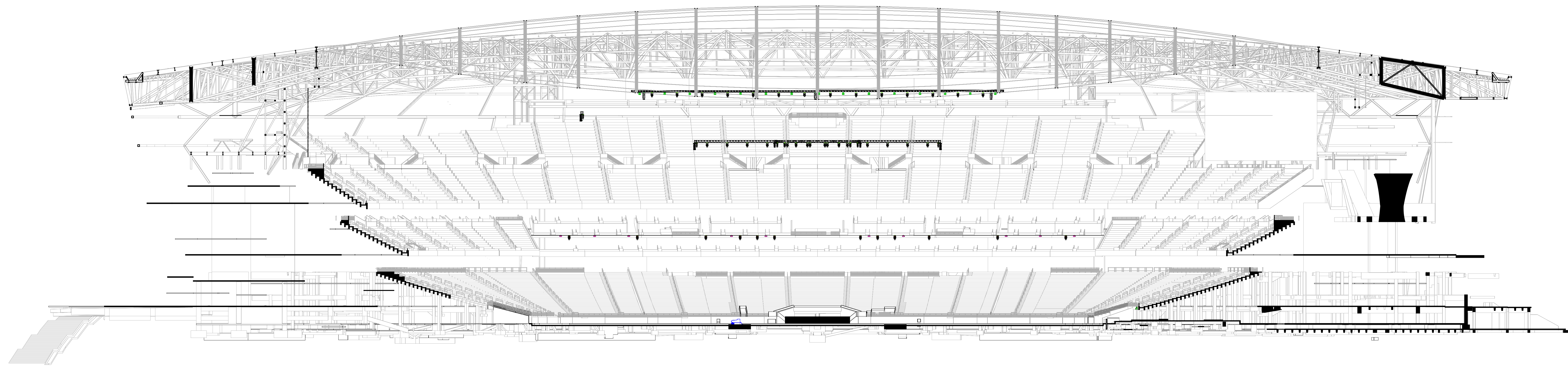
A SECTION DUE WEST Scale: 1" = 30'-0"
