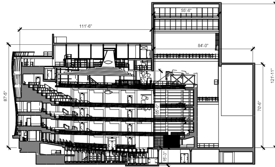
LONGITUDINAL SECTION
