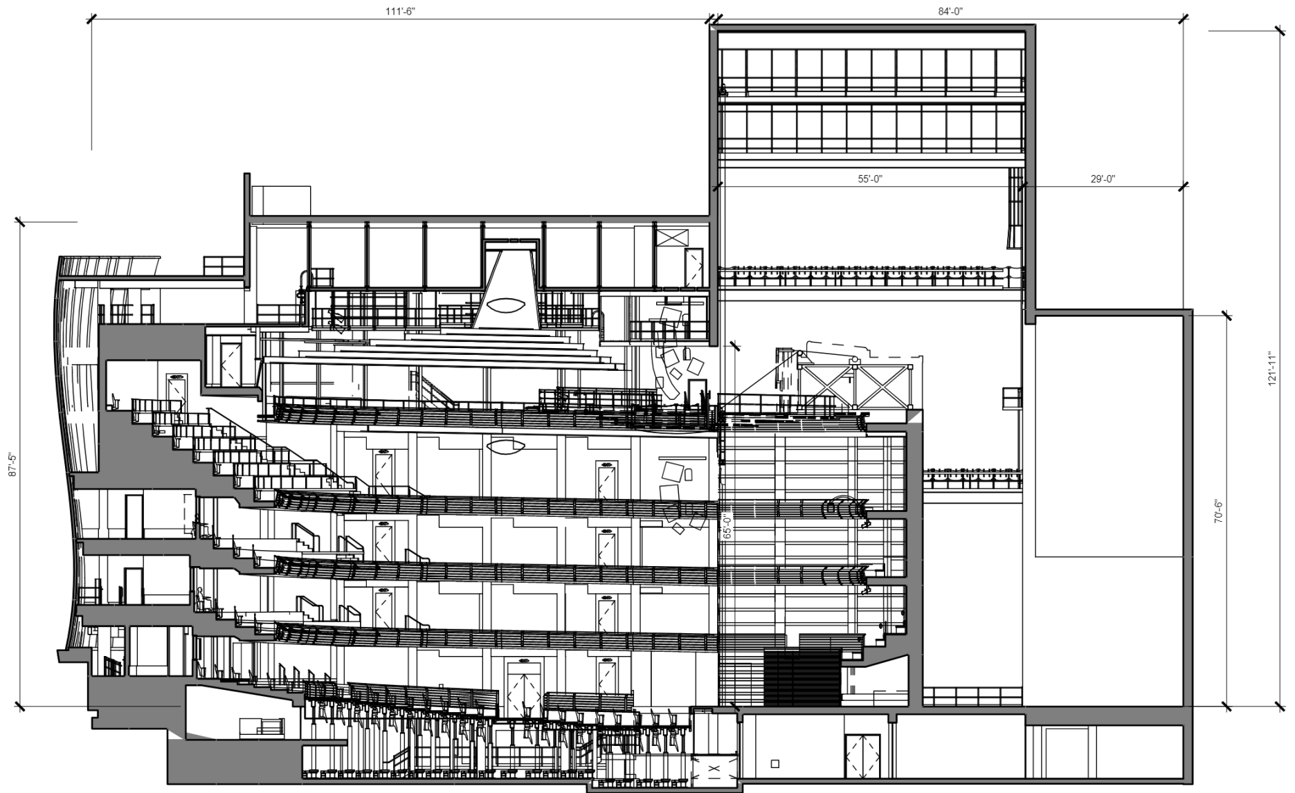
LONGITUDINAL SECTION
