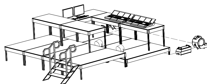
2 Isometric Scale: 1/2" = 1'-0"
