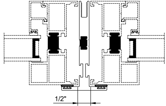
M24628 T-Mullion
