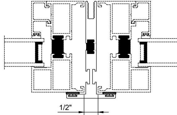
M24628 T-Mullion
