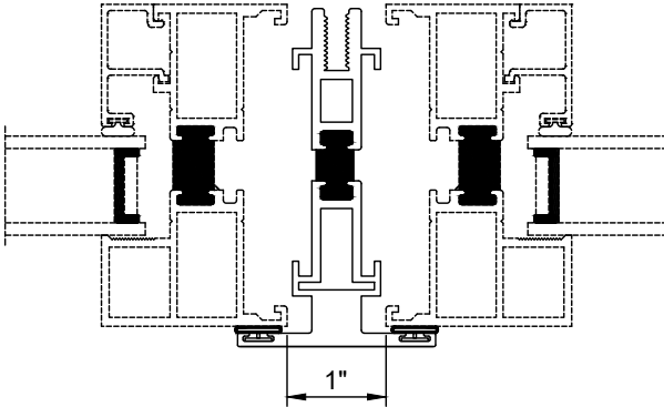
M22126 T-Mullion
