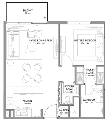
1 BEDROOM TYPE - 5
