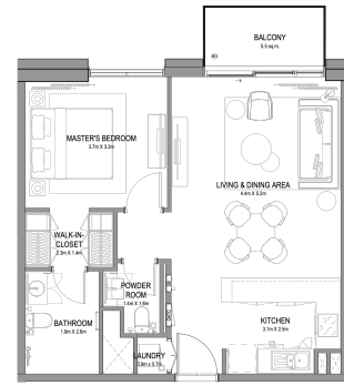
1 BEDROOM TYPE - 3
