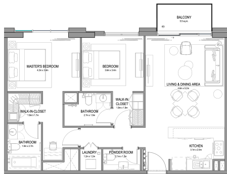
2 BEDROOMS TYPE - 3
