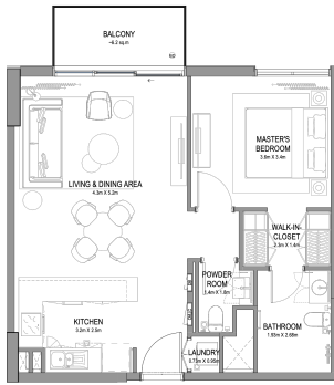
1 BEDROOM TYPE - 1
