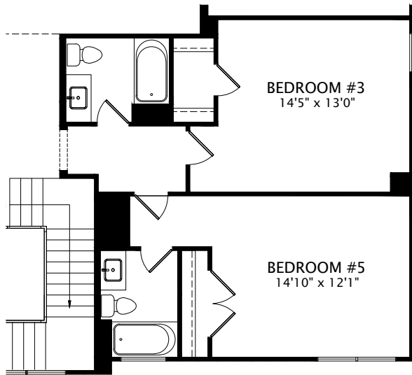
Optional Bedroom #5
