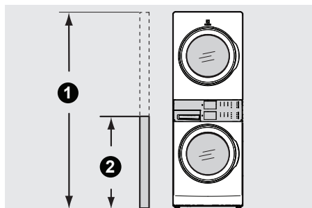
Las puertas bifoldables sólidas sin ventilación requieren la puerta abierta para 120 pulgadas cuadradas de ventilación en la pared
