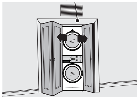
Las puertas bifoldables sólidas sin ventilación requieren la puerta abierta para 120 pulgadas cuadradas de ventilación en la pared
