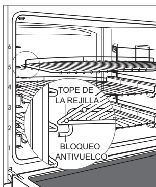
Bloqueo antivuelco para las rejillas del horno
