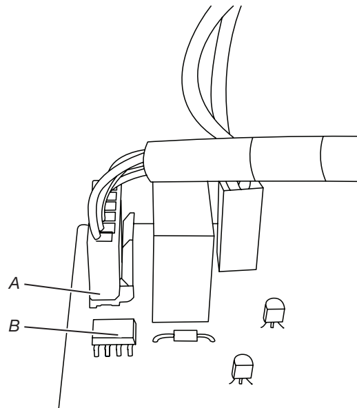
A. Arnés del extremo del conector blanco
