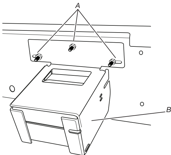
A. Écrous B. Lecteur de carte
