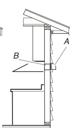
A. Wall cap B. 10" (25.4 cm) round vent
