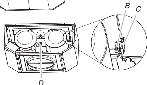
A. Couvercle avant B. Vis de montage du ventilateur C. Languette à ressort D. Prise électrique du moteur
