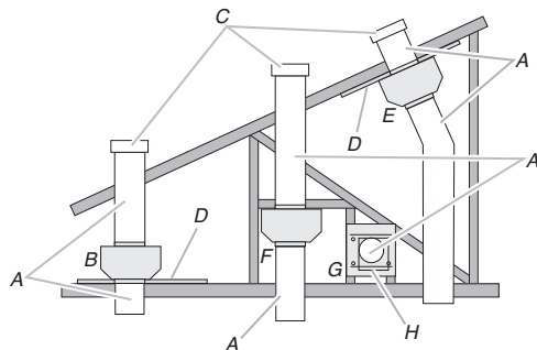
A. Conduit rond de 10 po (25,4 cm) B. Montage au-dessus des solives. C. Bouches de décharge sur toit D. Contre-plaqué (facultatif pour certaines installations) E. Montage sous les chevrons. F. Montage sur traverses de ferme. G. Conduit horizontal, montage sur traverses de ferme. H. Bouche de décharge murale
