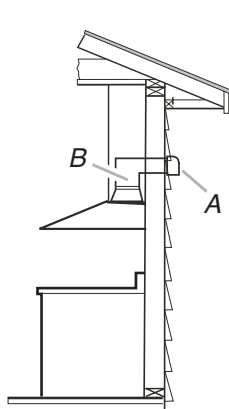
A. Wall cap B. 10" (25.4 cm) round vent
