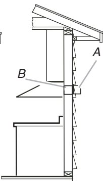
A. Bouche de décharge murale B. Conduit rond de 10 po (25,4 cm)
