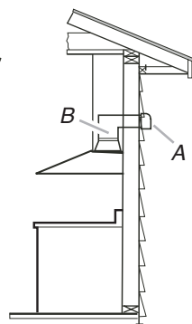
A. Bouche de décharge murale B. Conduit rond de 10 po (25,4 cm)
