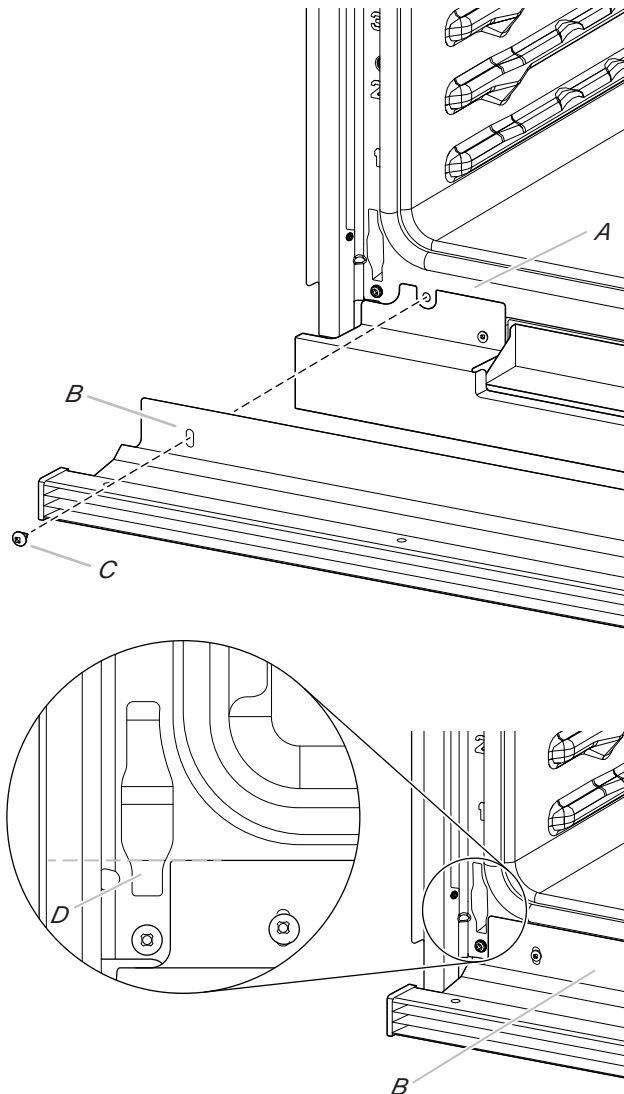
A. Marco del horno C. Tornillo n.º 8-18 x 3/8" (9,5 mm) B. Lengüeta de ventilación D. Receptor de bisagra
