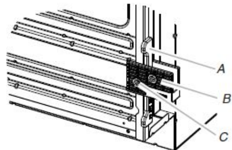
A. Espaciador B. Pata C. Tornillo n.º 8-18 x 3/8" (9,5 mm)
