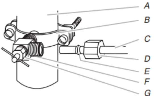
A. Canalisation d'eau froide B. Bride de tuyau C. Tube de cuivre D. Écrou de compression E. Virole de compression F. Robinet d'arrêt G. Écrou de presse-étoupe
