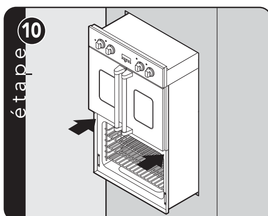
Poussez le four droit dans son logement.
