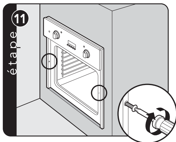
Posez des vis sur le côté du châssis. Remarque: 3 vis pour les fours simples, 4 pour les doubles (vis non fournies)
