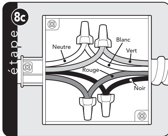
Option de câblage 3* (branchez le blanc sur le neutre d'arrivée, et le vert sur une terre convenable)
