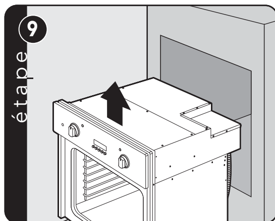
Levez le four en position.
