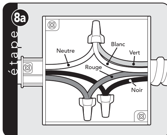
Option de câblage 1* (branchez blanc et vert sur le neutre d'arrivée)
