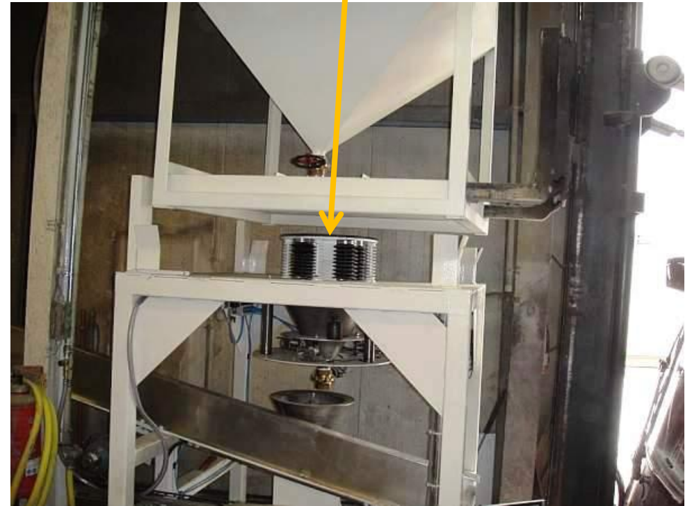
Druckplatte zum Andocken des Behälters auf das Grundgestell
