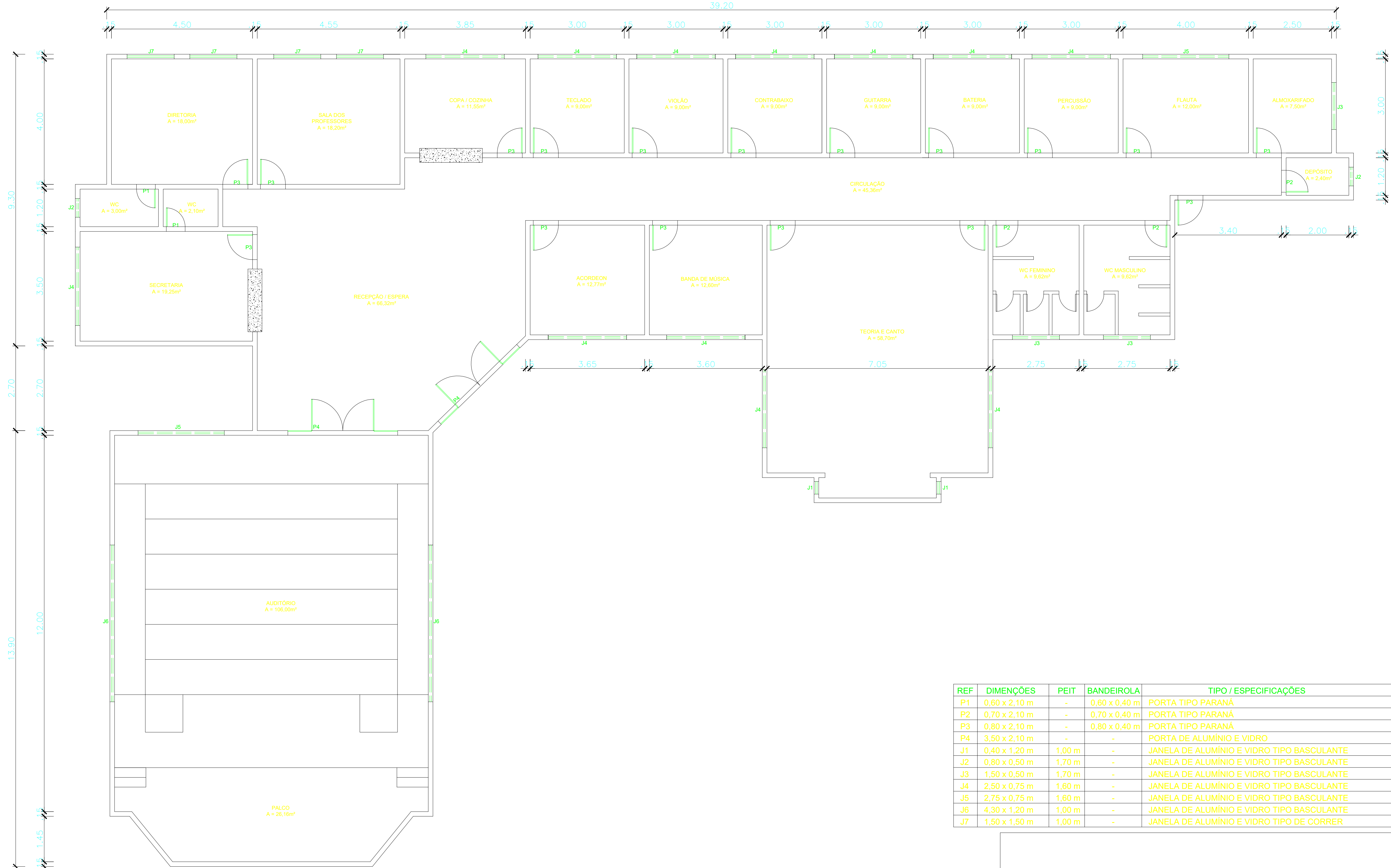
01 PLANTA BAIXA ESC. 1/100
