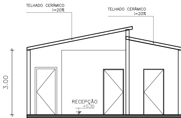
CORTE AA ESC. 1:100
