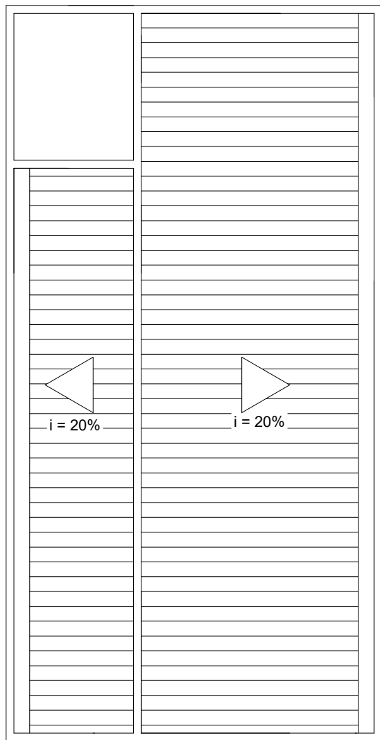
PLANTA DE COBERTA ESC. 1:100
