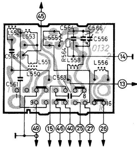
Fig. 25 PL 5 (PT 4079/2..z) Bedruckungsseite/printed side
