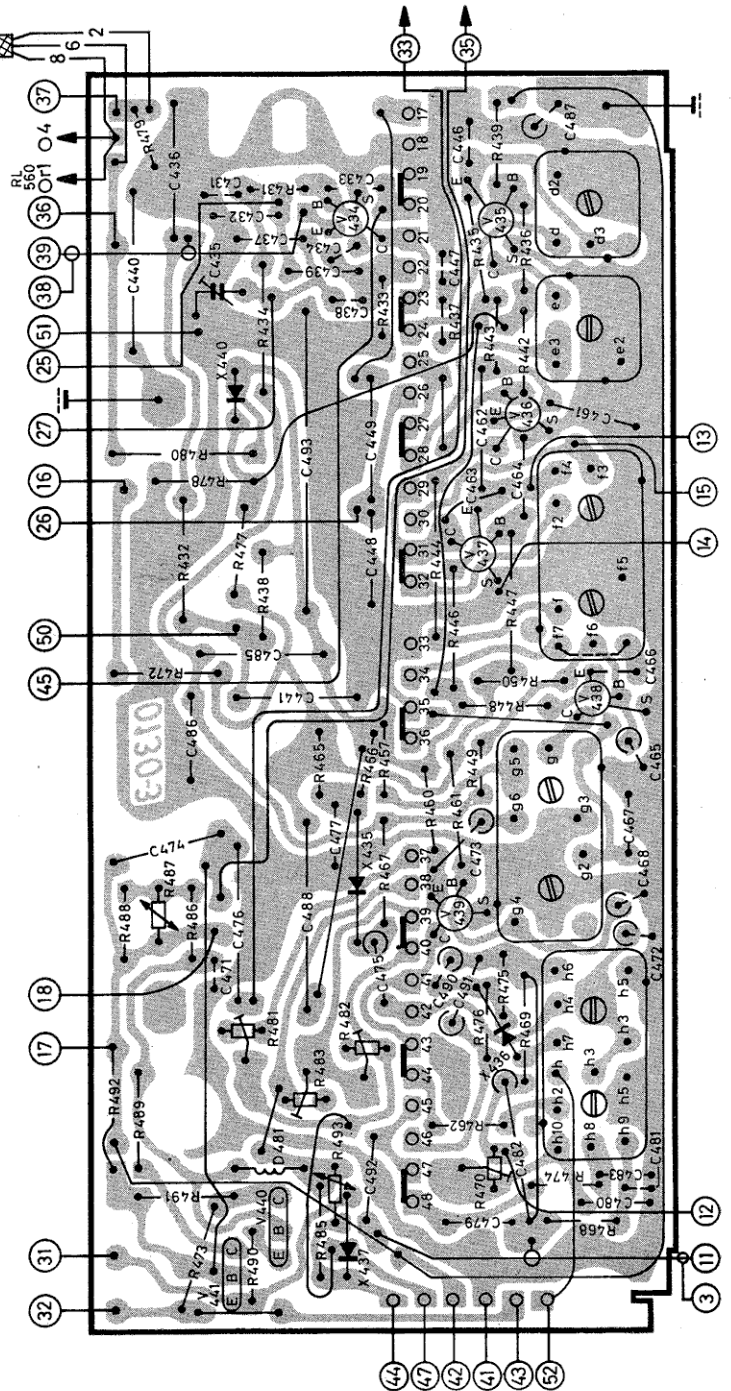
Fig. 26 PL 3 (PT 4078/3..z) Bestückungsseite/components side
