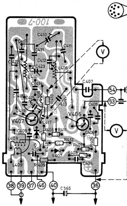
Fig. 24 PL 4 (PT 4072/4..z) Bedruckungsseite/printed side
