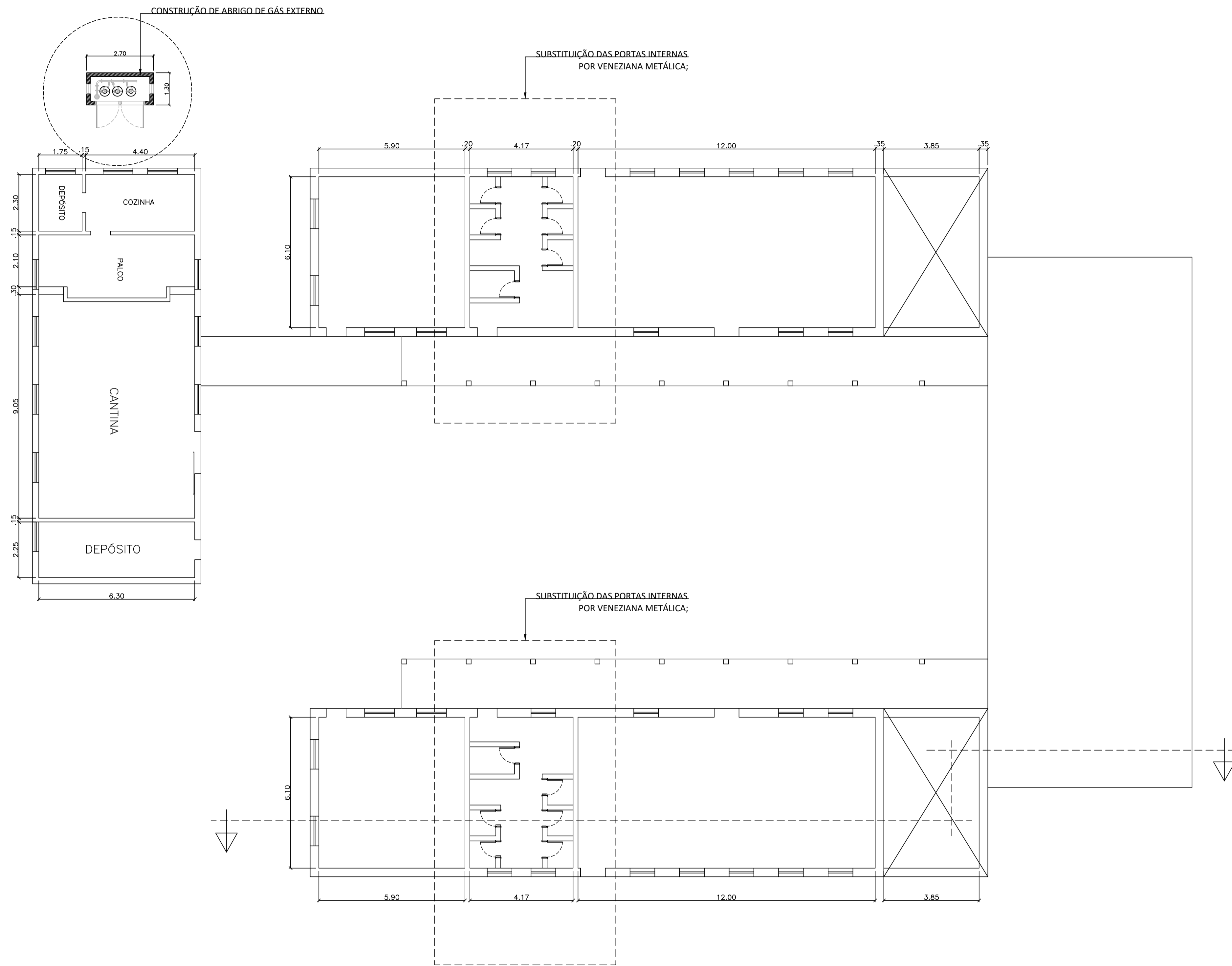
PLANTA BAIXA - PROJETO REFORMA ESCOLAR - SUBSOLO esc 1:100
