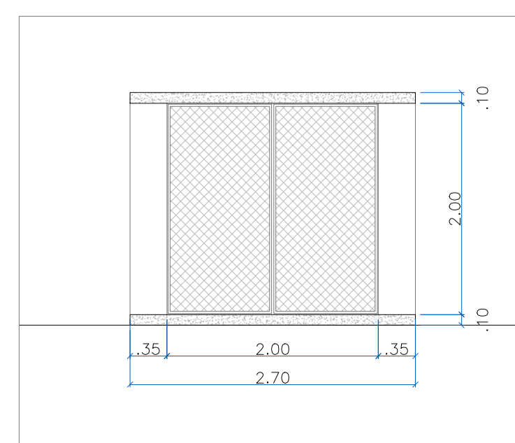
ABRIGO DE GÁS SEM ESCALA
