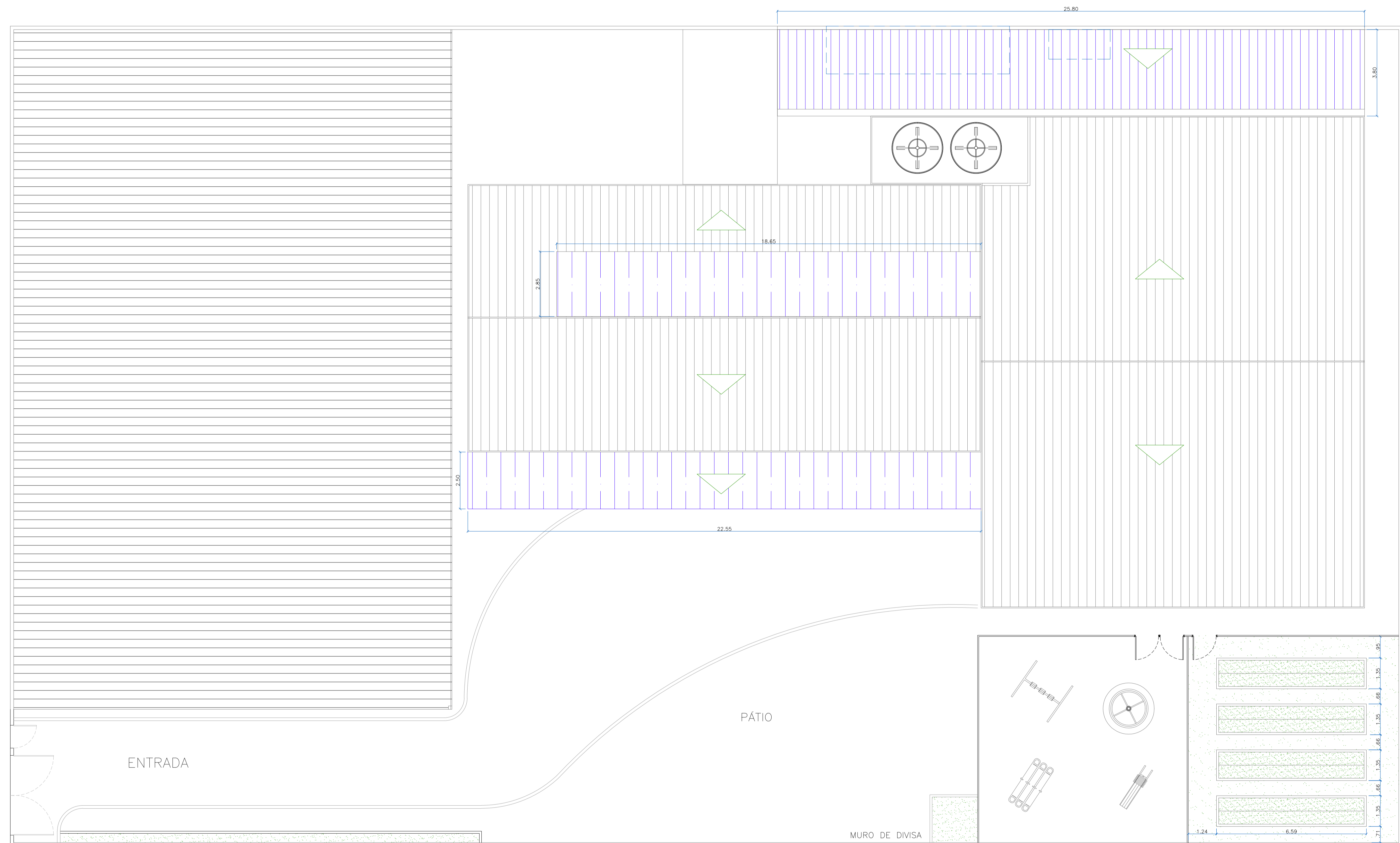
PLANTA DE COBERTURA - PROJETO REFORMA ESCOLAR esc 1:100
