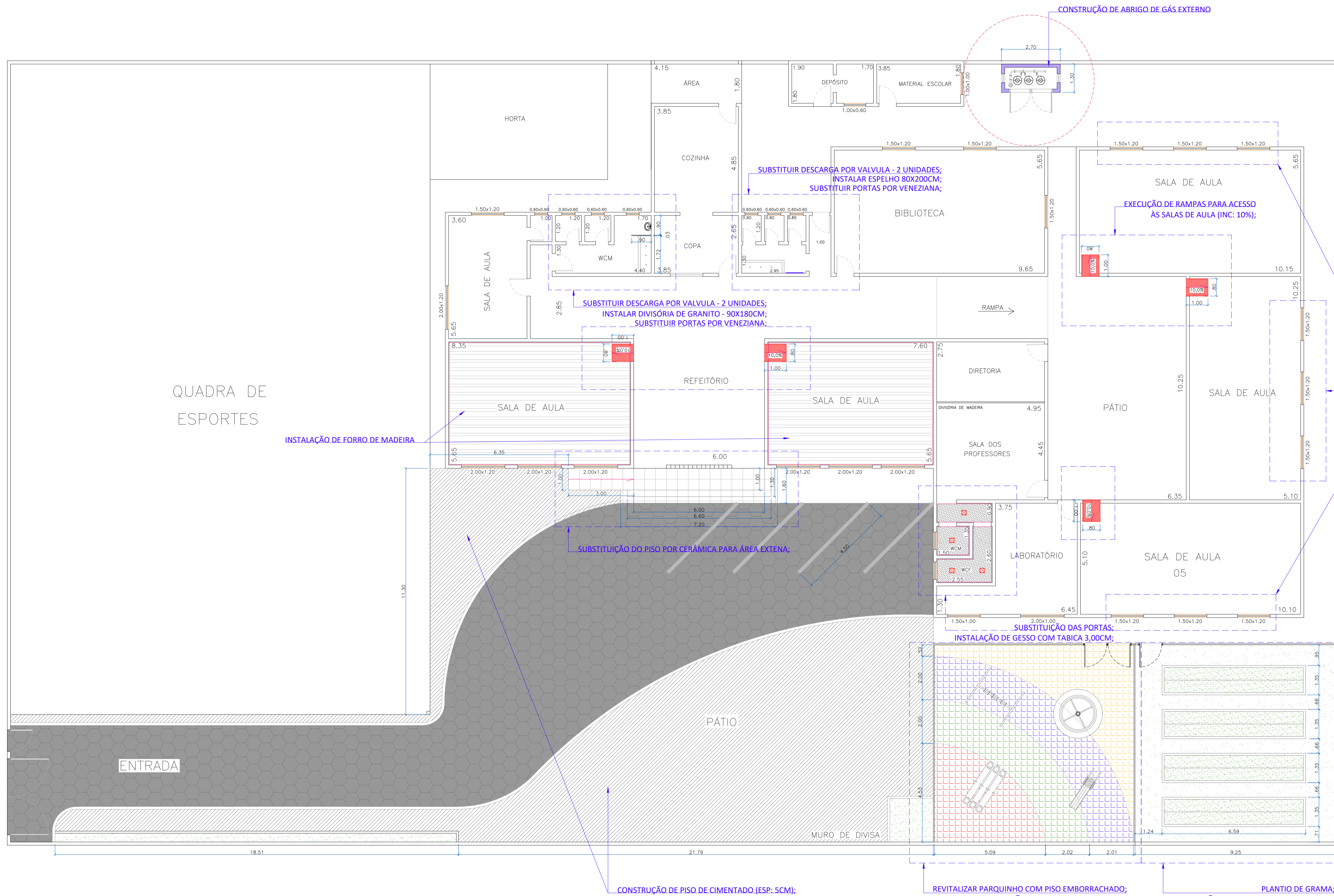
PLANTA BAIXA - PROJETO REFORMA ESCOLAR esc: 1:100
