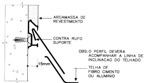
ARREIMATE DE LATERAL DE TELHADO COM PAREDE. INSTALACAO ALINHADA PELO REVESTIMENTO
