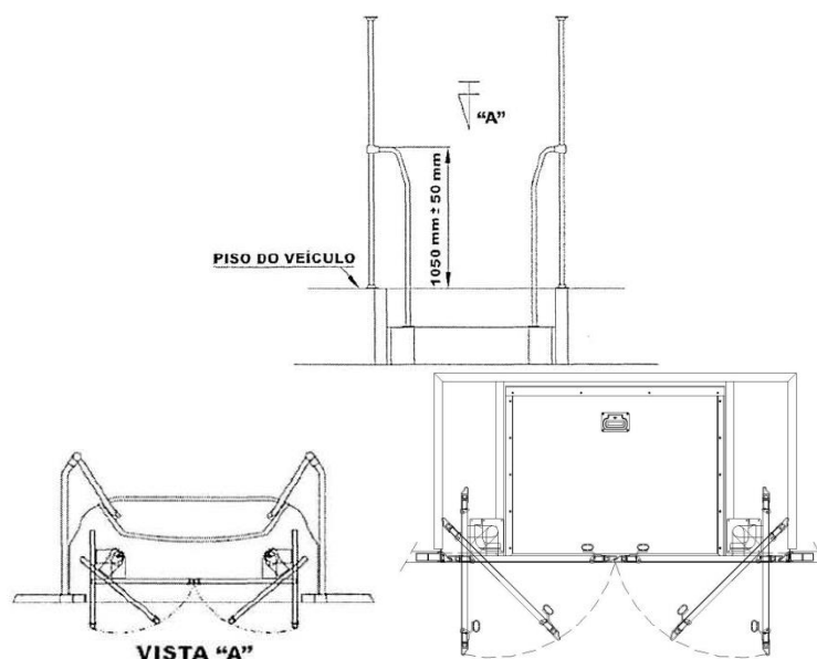
Figura 06 – Imagem ilustrativa: instalação dos corrimãos inferiores
