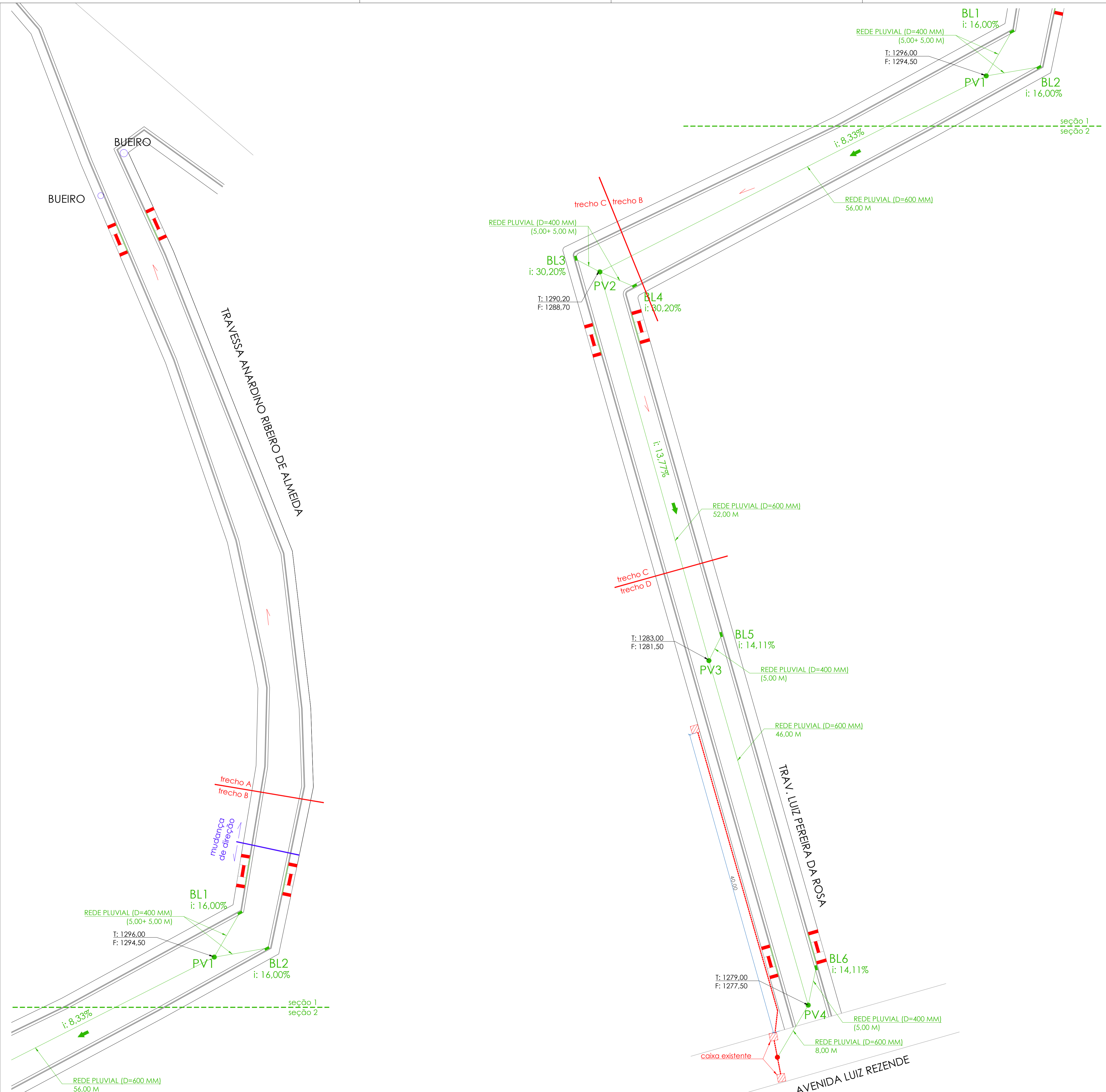
TRAV. LUIZ PEREIRA DA ROSA E TRAV. ANARDINO RIBEIRO DE ALMEIDA- DRENAGEM (seção 1) ESCALA 1/250
