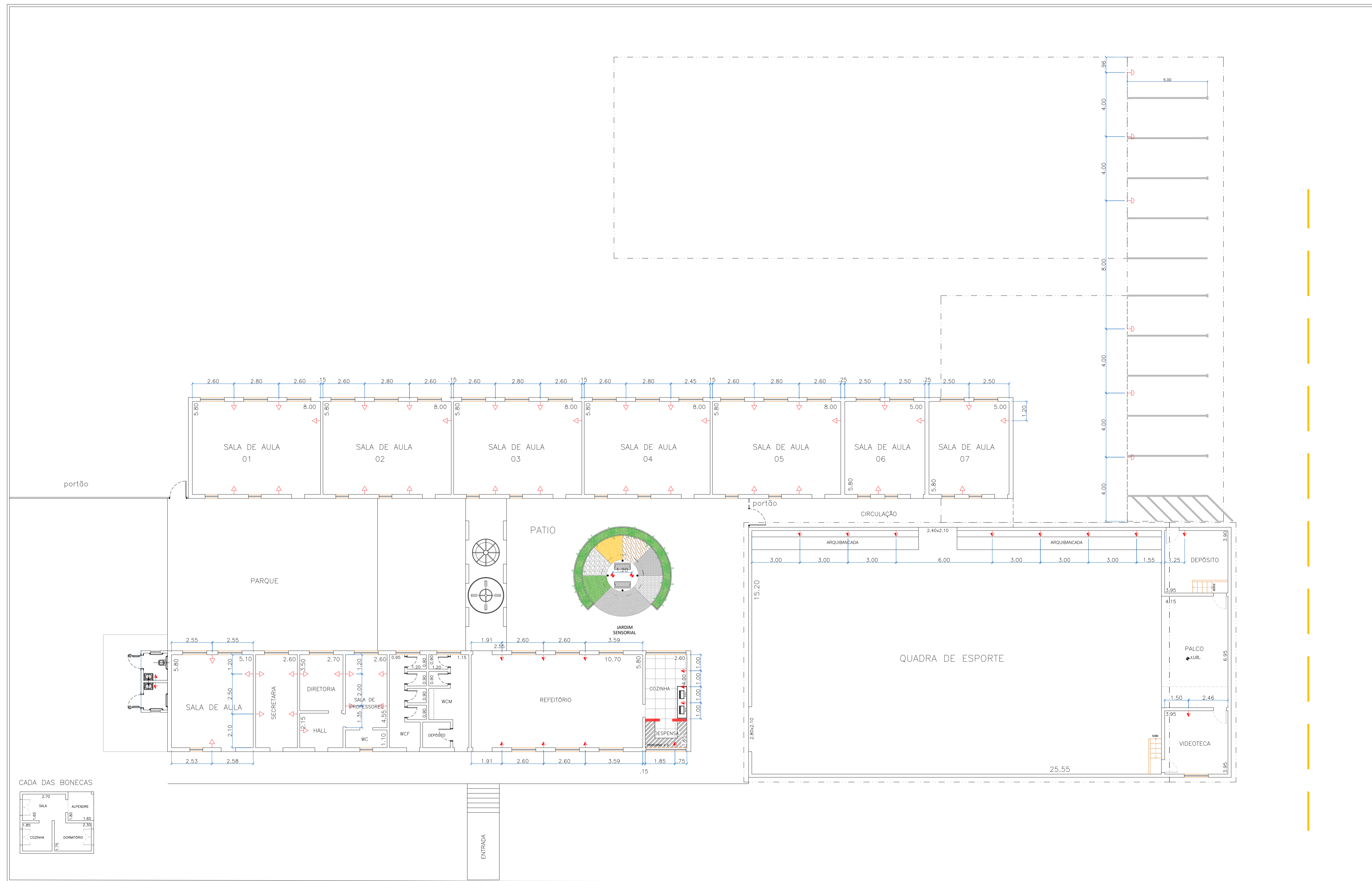
PLANTA BAIXA - INDICAÇÃO DE PONTOS ELÉTRICOS - REFORMA ESCOLA TIA EMILIA esc. 1:125
