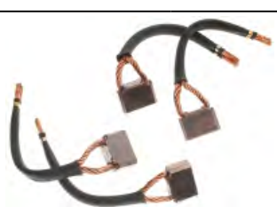
E500 Alternator / Generator Brush Set TAB 127; 1004 320 031; CE 11057
