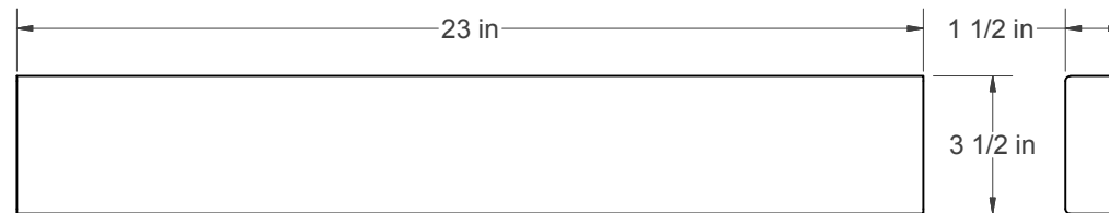
(D) - LONG CROSS RAILS (MAKE TWO)
