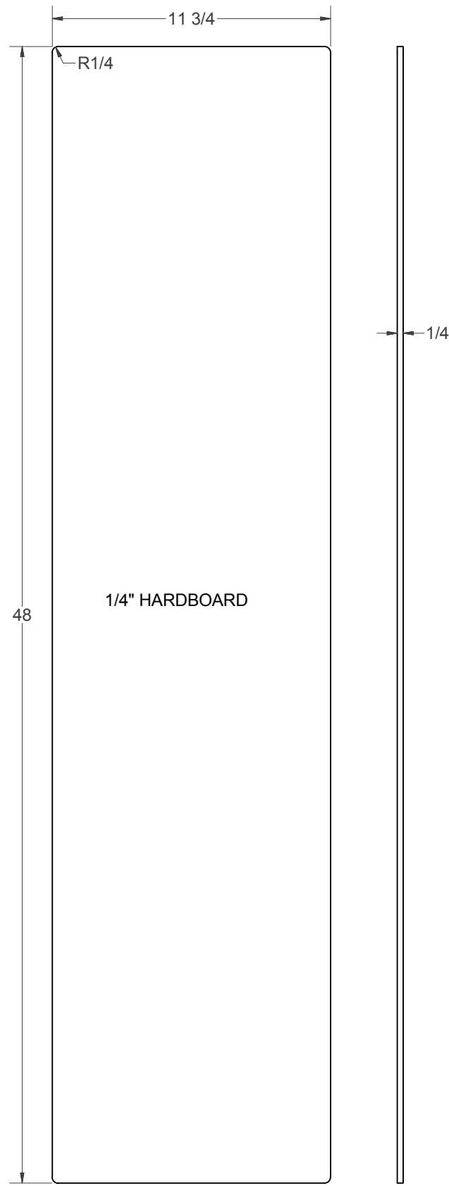
A - BOTTOM (1)
