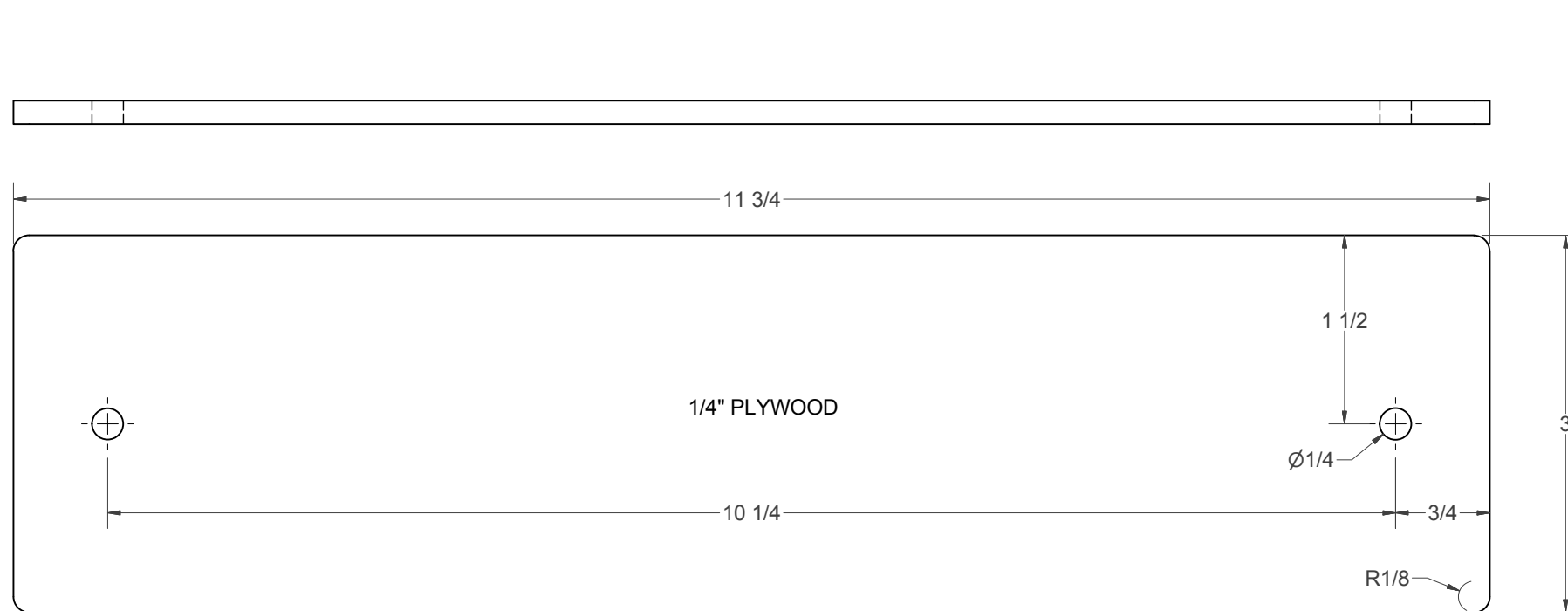
F - BASEPLATE (5)
