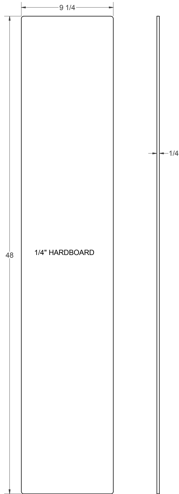
D - TOP (1)
