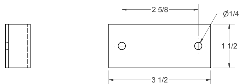
(V) - TOOL CLAMP
