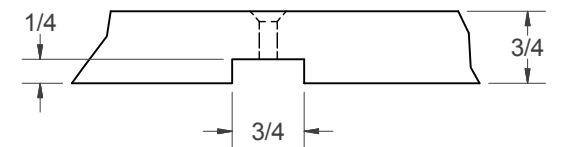
DIVIDER PANEL DADO
