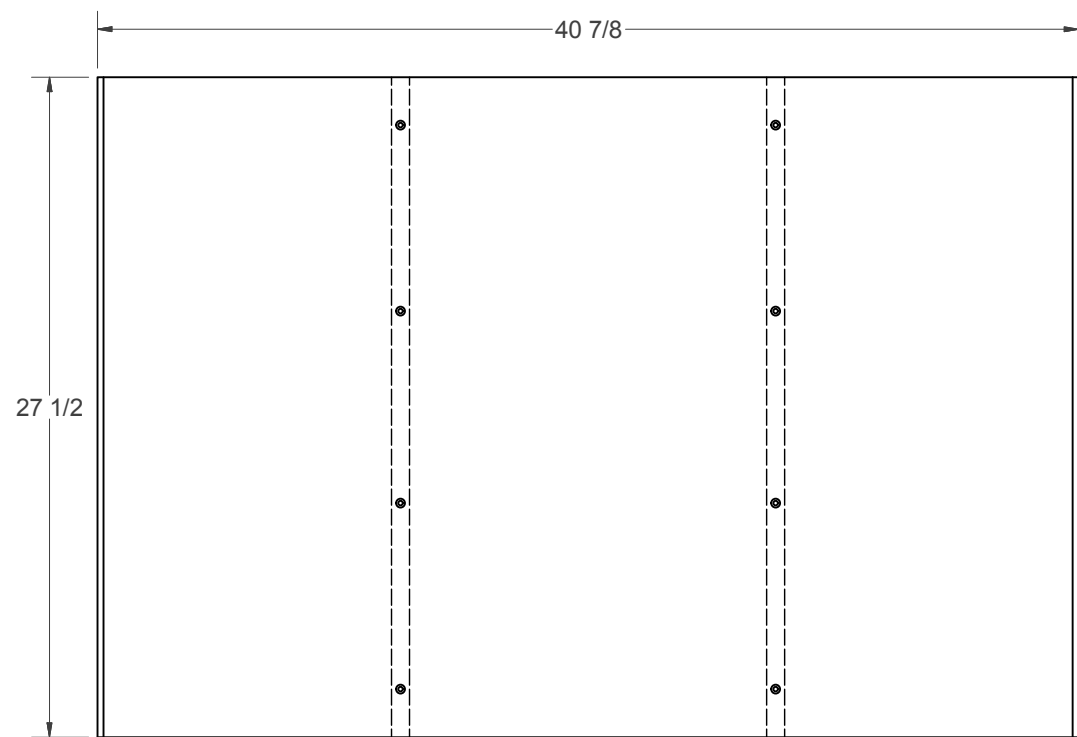
(N) - CASE BOTTOM
