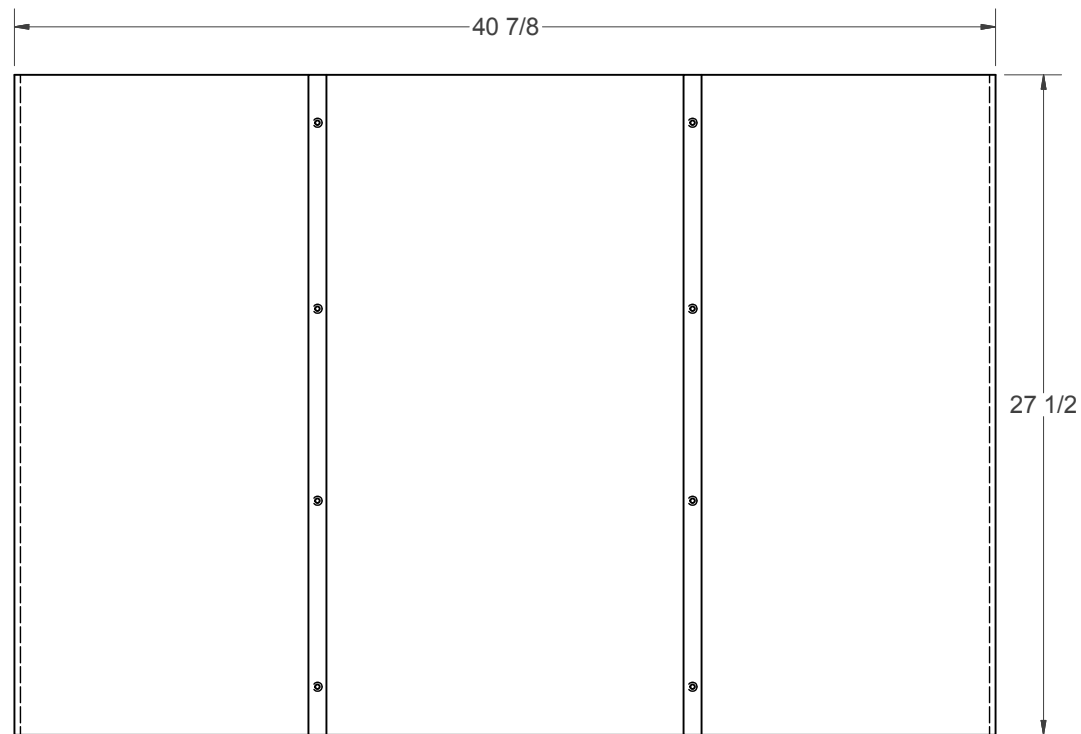
(N) - CASE TOP
